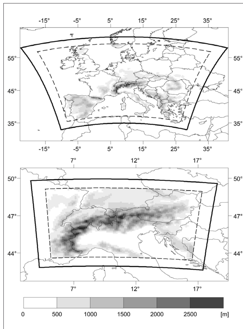
Fig. 5.8: Spatial MM5 setup. Upper panel: intermediate model domain (30 km × 30 km grid spacing). Lower panel: high resolution model domain (10 km × 10 km grid spacing). The grey scales indicate the model orography. Räumliche MM5 Konfiguration. Obere Abbildung: Modellgebiet 1 (30 km × 30 km Gitterpunktsabstand). Untere Abbildung: Modellgebiet 2 (10 km × 10 km Gitterpunktsabstand). Die grauen Schattierungen zeigen die Modell-Orographie.
