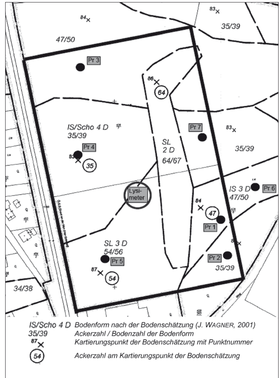
Fig. 5.6: Finanzbodenschätzung – Reinkarte (J. WAGNER, 2001) des Versuchsfeldes Wagner mit den Profilstellen Pr 1 bis Pr 7, der Lage des Lysimeterstandortes und der Umgrenzung des Großpartzellenversuchs Wagner. Soil map (J. WAGNER, 2001) of the agricultural test field Wagner with soil profiles Pr 1 to Pr 7, the lysimeter station and the border of test area.
