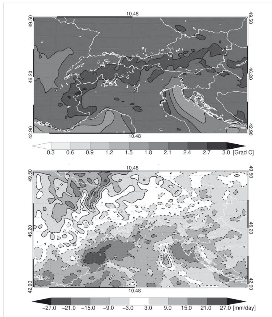
Fig. 5.9: Annual mean differences between the MMS scenario (2041 to 2050) and control (1981 to 1990) simulation. Upper panel: temperature change [°C], lower panel: precipitation change [mm/day]. Mittlere jährliche Änderung zwischen der Szenario- (2041 bis 2050) und der Kontrollsimulation (1981 bis 1990). Obere Abbildung: Temperaturänderung [°C]. Untere Abbildung: Niederschlagsänderung [mm/Tag].
