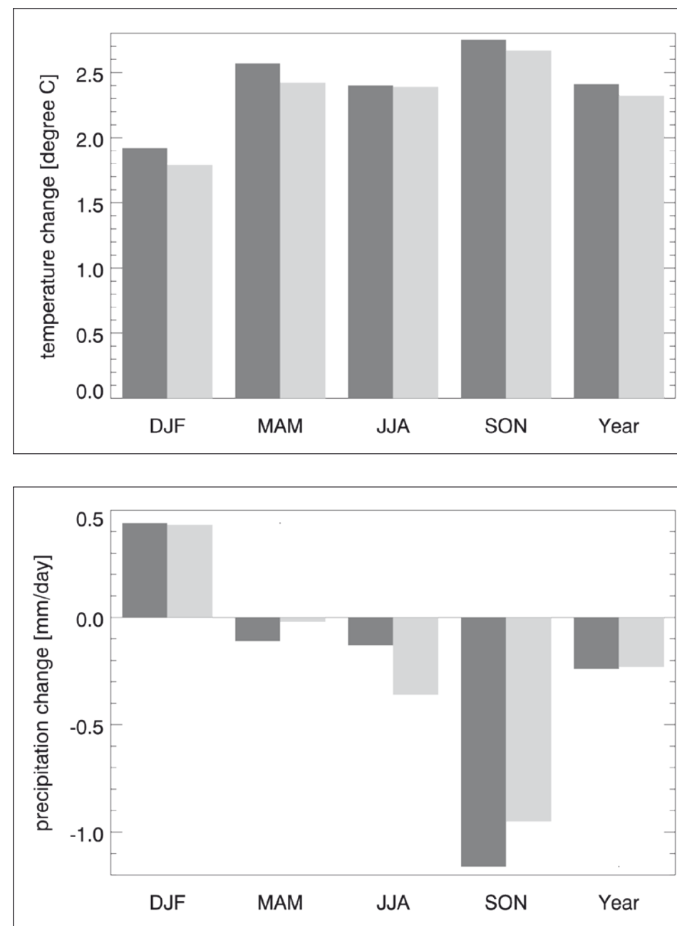
Fig. 5.10: Seasonal differences between the scenario (2041 to 2050) and control (1981 to 1990) simulation in south-eastern Styria. Mountainous part: dark grey, hilly part: light grey. Upper panel: temperature change [°C], lower panel: precipitation change [mm/day]. Saisonale Änderung zwischen der Szenario- (2041 bis 2050) und der Kontrollsimulation (1981 bis 1990) in der Südoststeiermark. Gebirgiger Teil: dunkelgrau, hügeliger Teil: hellgrau. Obere Abbildung: Temperaturänderung [°C]. Untere Abbildung: Niederschlagsänderung [mm/Tag].
