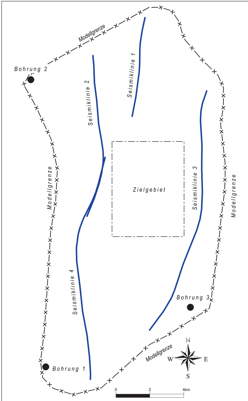
Fig. 2: Untersuchungsgebiet Puchheim-Germering. Geophonversenkmessungen liefern für bekannte Tiefen eine seismische Laufzeit. Aus diesen so genannten Zeit-Tiefen-Paaren kann man Geschwindigkeitsinformationen ableiten.
